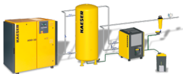
Druckluft-Aufbereitung (Filter, Kondensat-Aufbereitung, Adsorptionstrockner, Aktivkohleadsorber)
